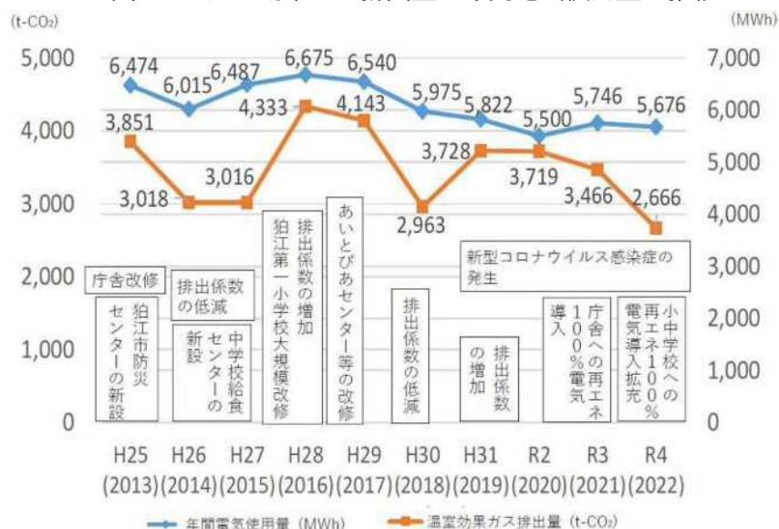
図6-1 温室効果ガス排出量と年間電気使用量の推移
