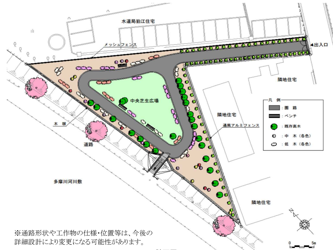
計画図
