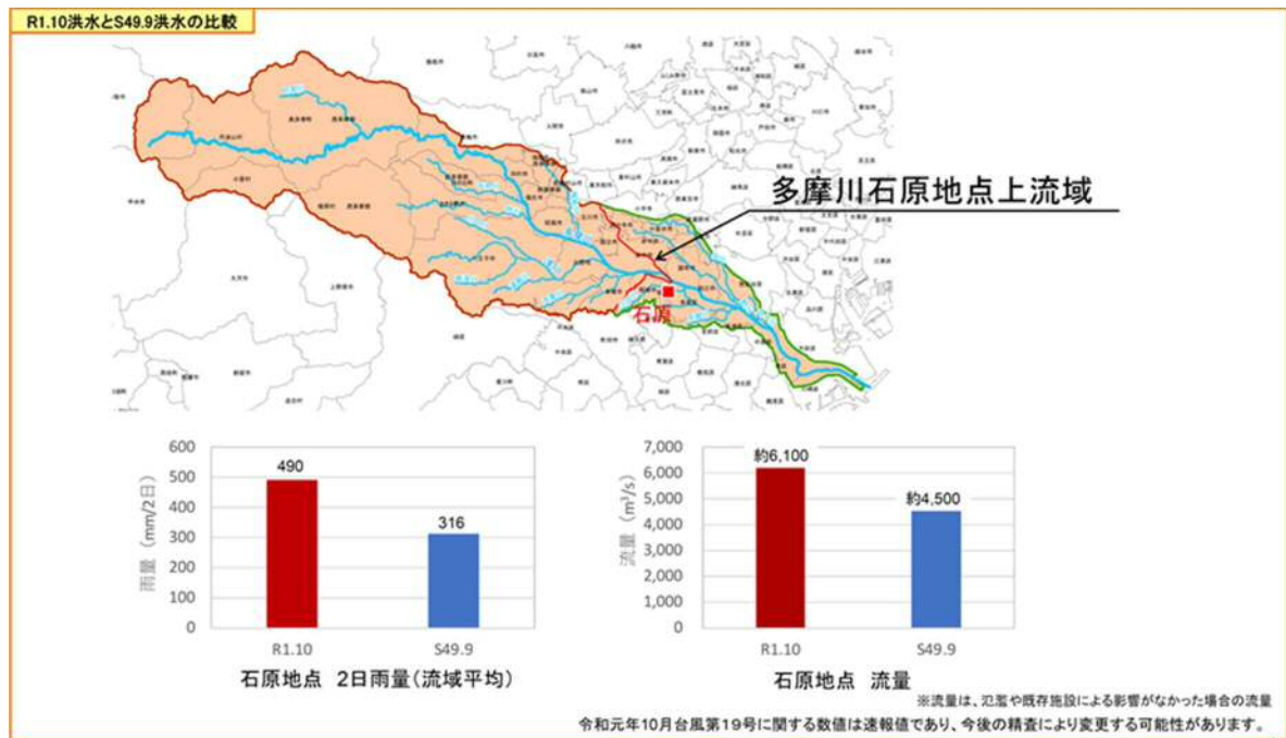
図 2-2-2 今回洪水(令和元年 10 月洪水)と現行整備計画目標洪水(昭和 49 年 9 月洪水)
