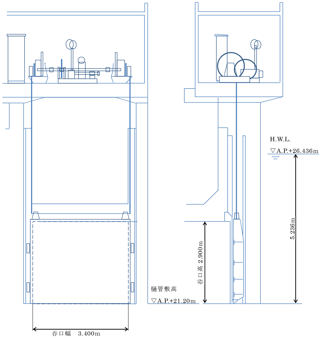
図 3-3-4 ゲート構造図 (六郷排水樋管)
