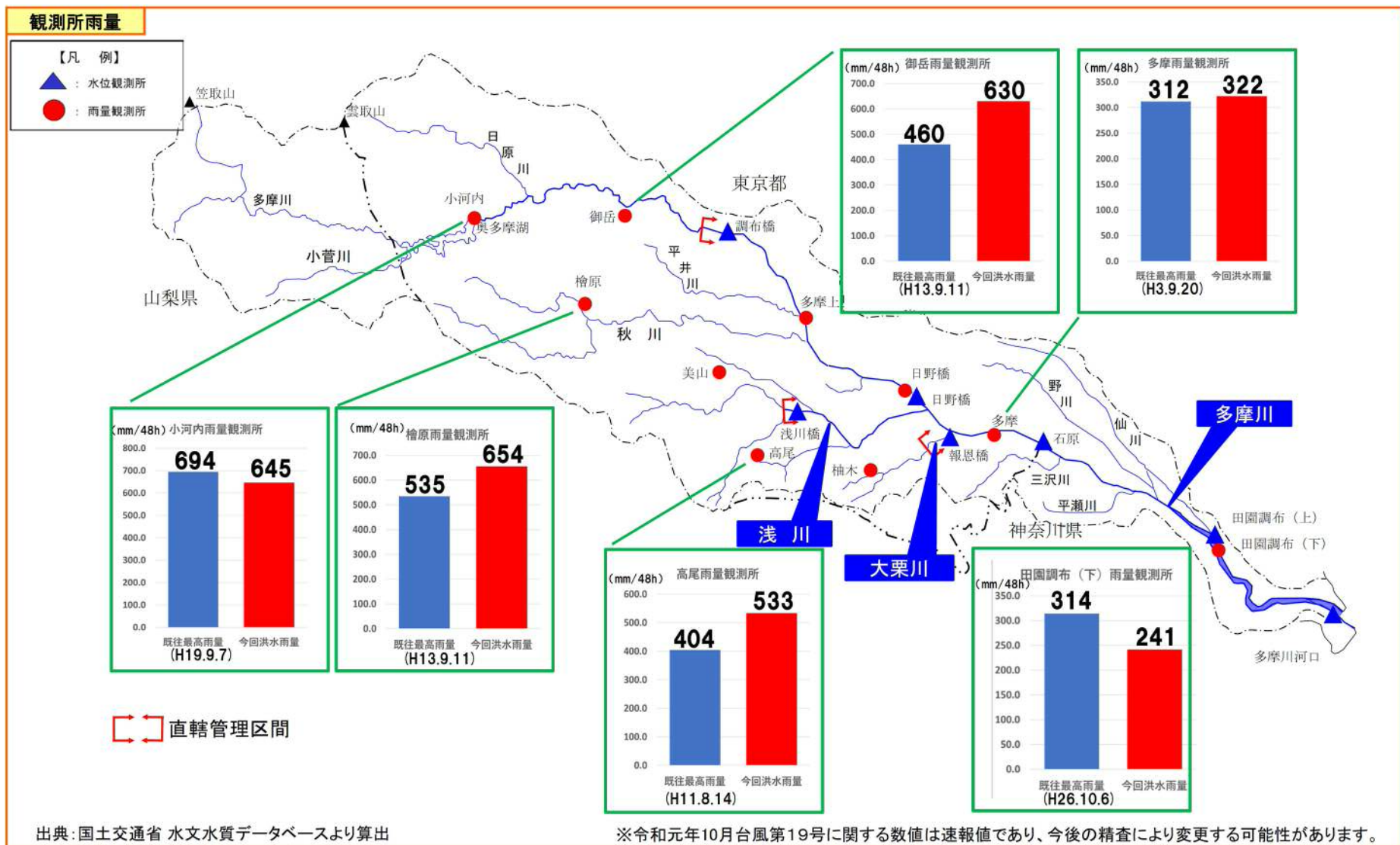
図 2-2-1 多摩川流域の雨量・水位観測所と雨量
