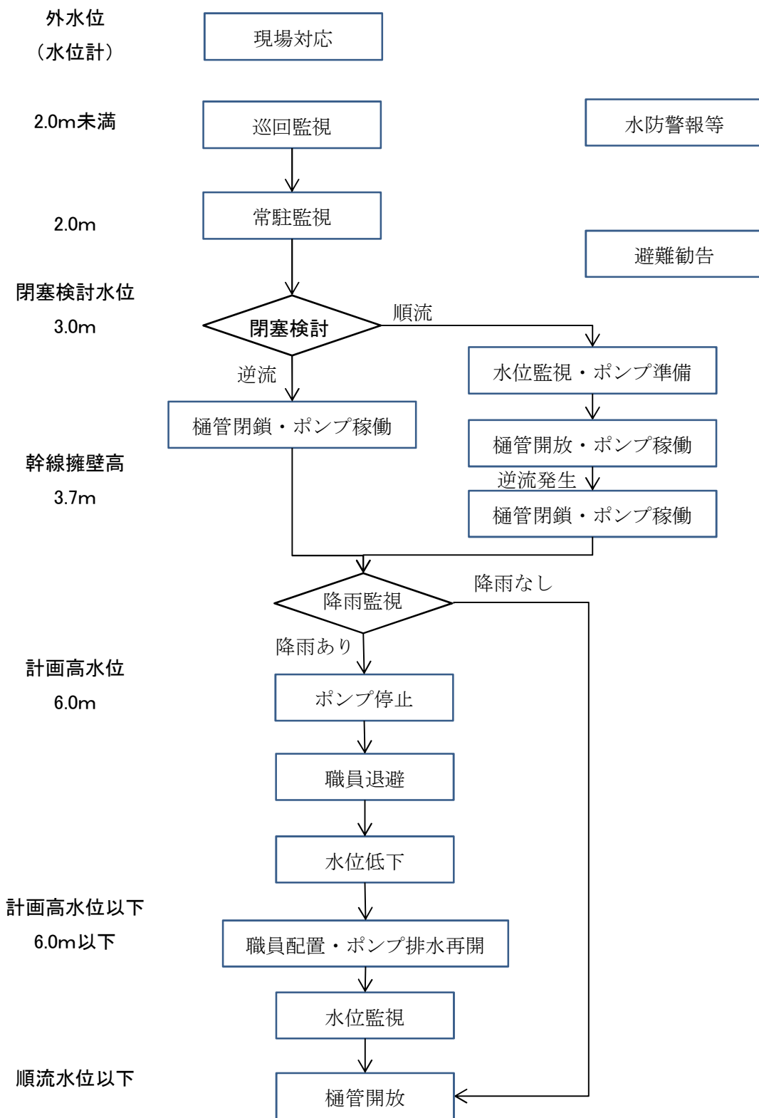
図 6-1-1 操作フロー案 (六郷排水樋管)
