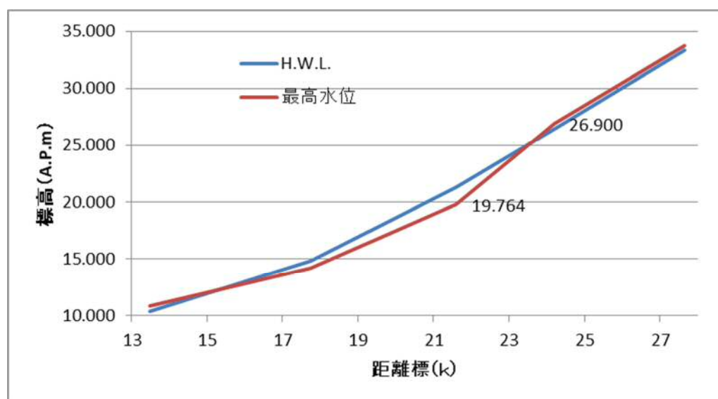
図 5-2-1 H.W.L. と最高水位縦断図
