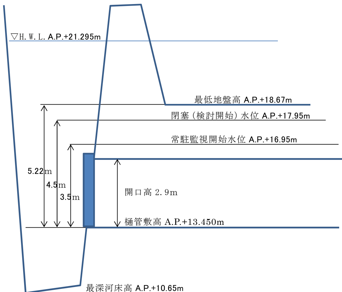
図 4-2-2 猪方排水樋管の高さ関係整理
