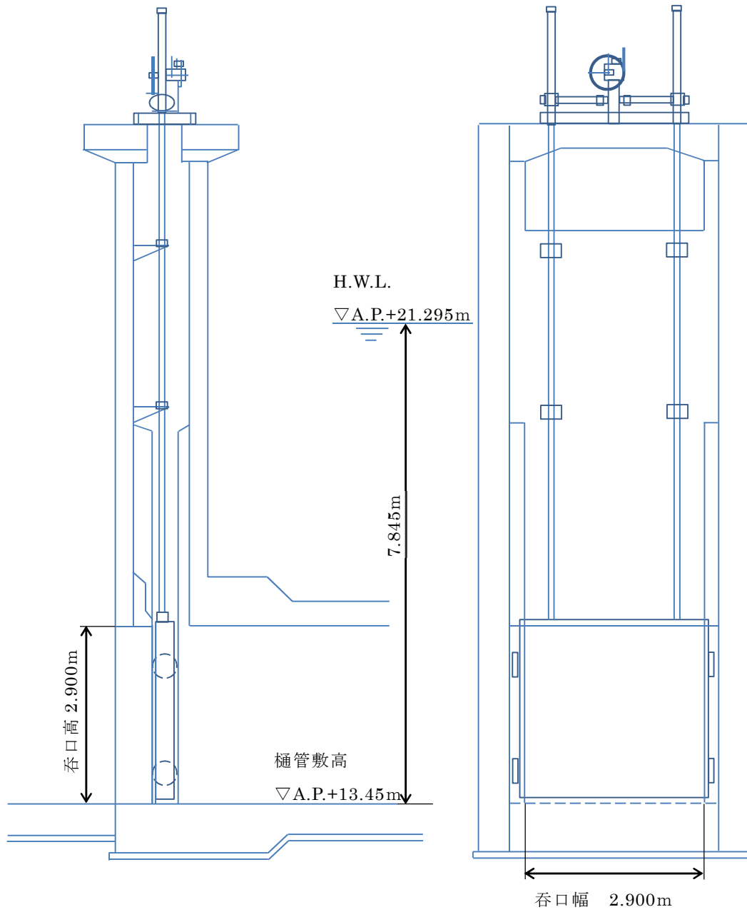
図 3-3-2 ゲート構造図 (猪方排水樋管)
