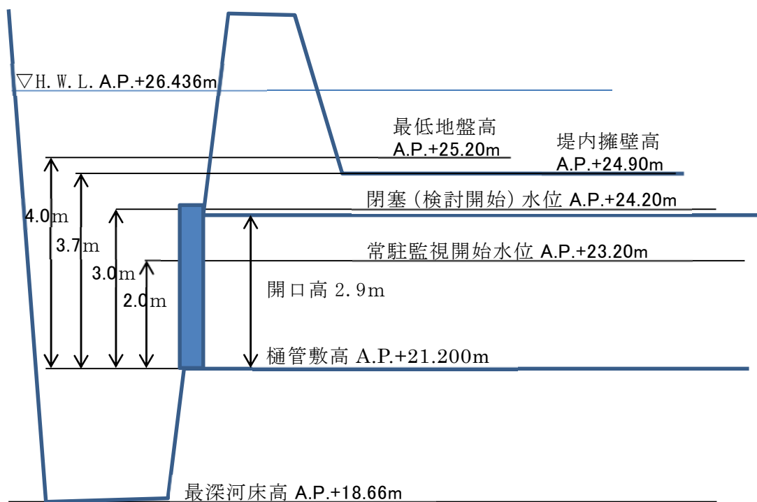
図 4-2-4 六郷排水樋管の高さ関係整理
