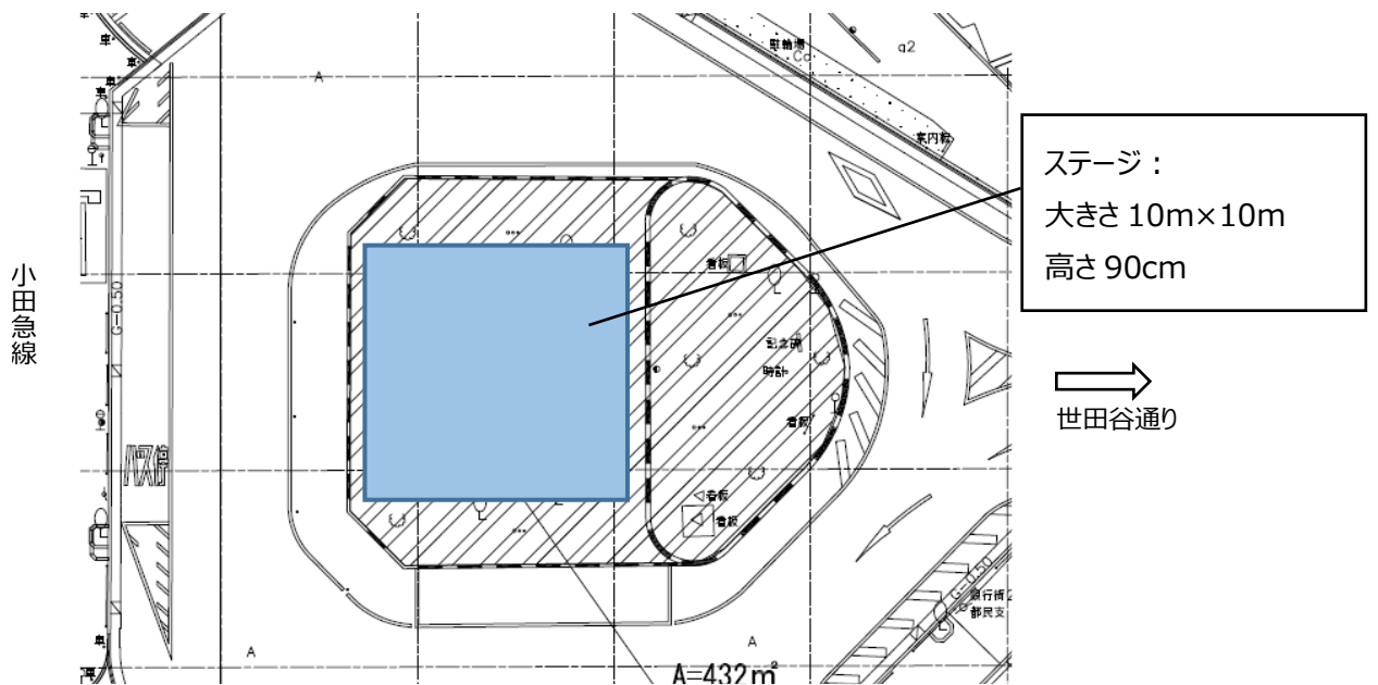
ステージ施工予定図：
