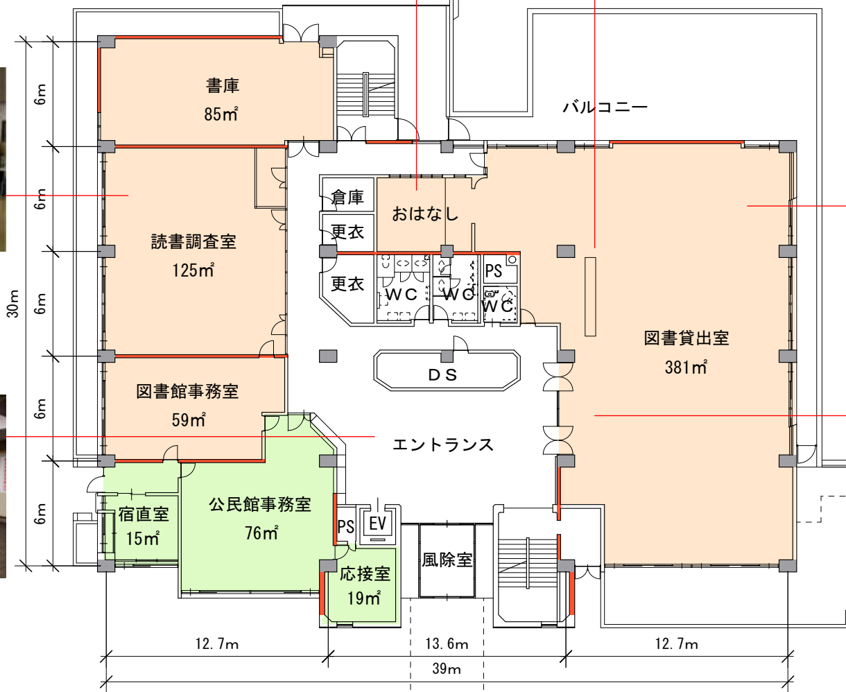
既存1階平面図 S=1:300
