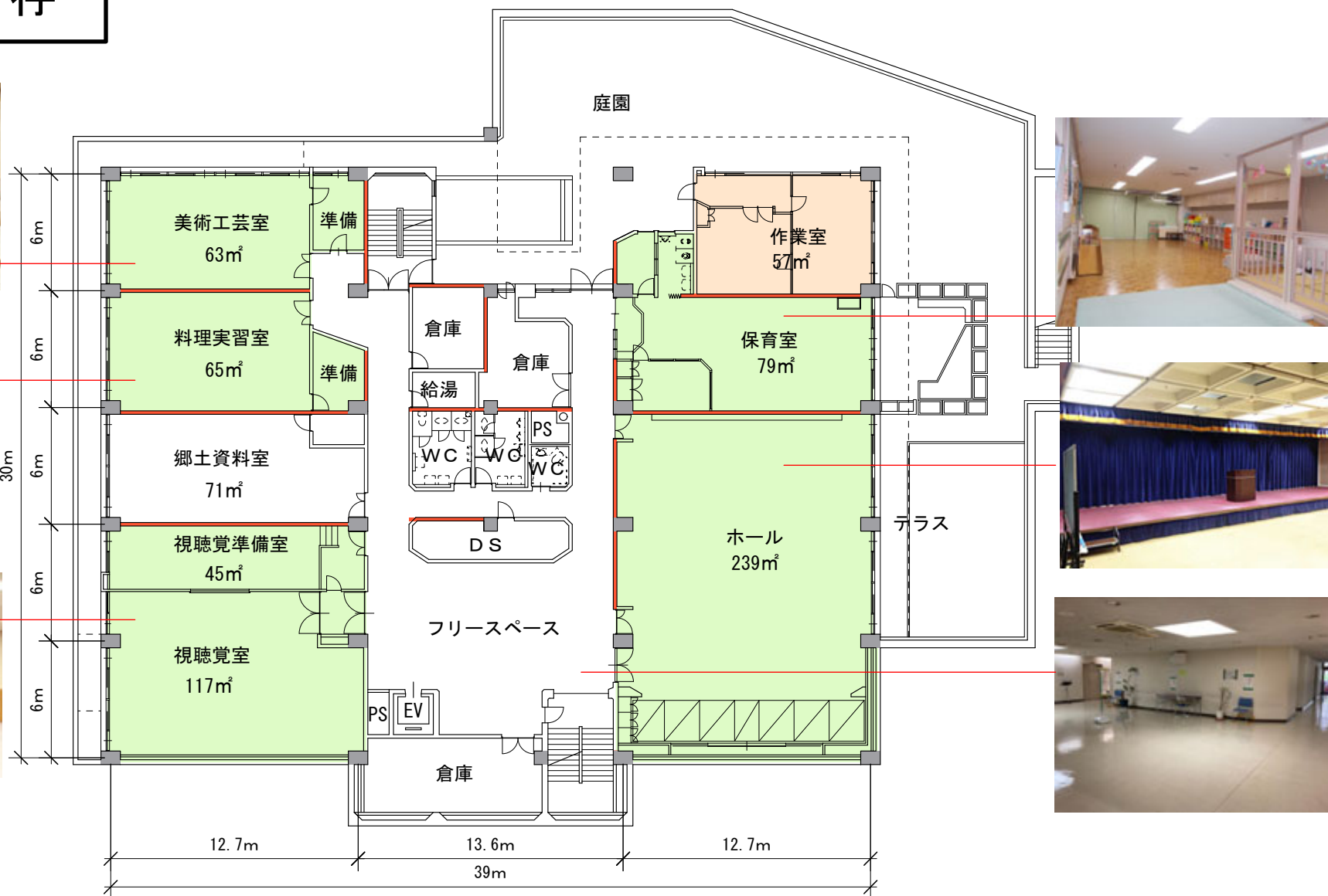
既存地下1階平面図 S=1:300
