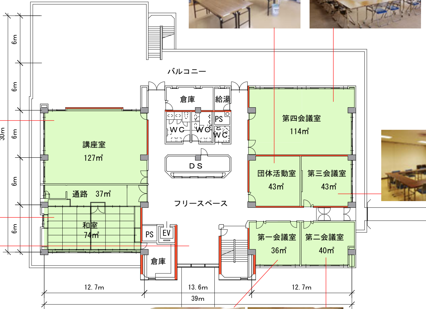
既存 2階平面図 S=1:300
